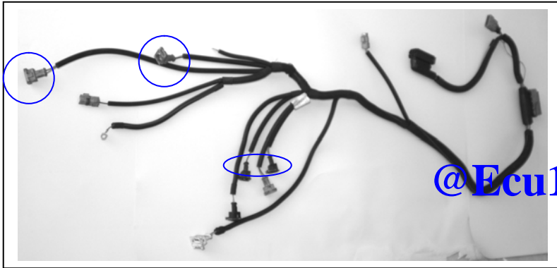
دسته سیم جدید موتور (سریال ۶۰۳۰۵۲) که سوکتهای اضافی آن در شکل مشخص شده است .
