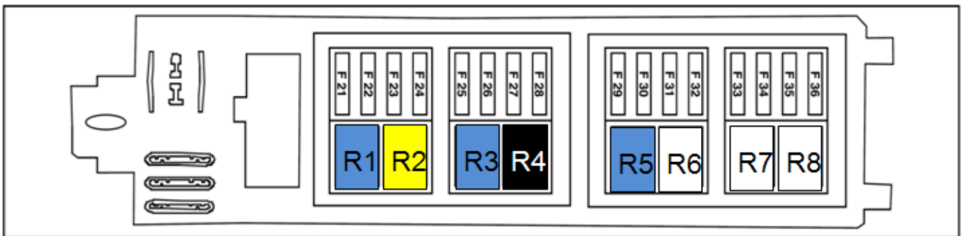
جدول راهنمای فیوزهای داخل اتاق (BCM) @Ecu118
